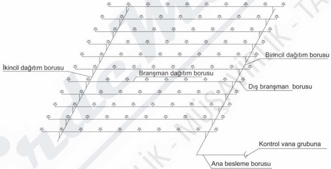
Şekil 7.2.3 Grid Borulama Sistemi
