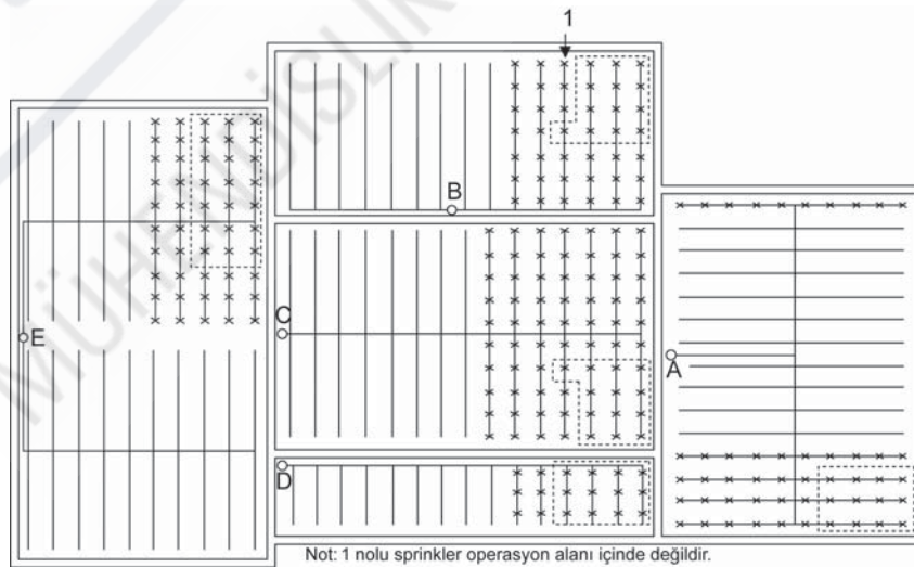
Şekil 7.4.3.2 (b) Kritik Hidrolik Tasarım Alanı Örnekleri
