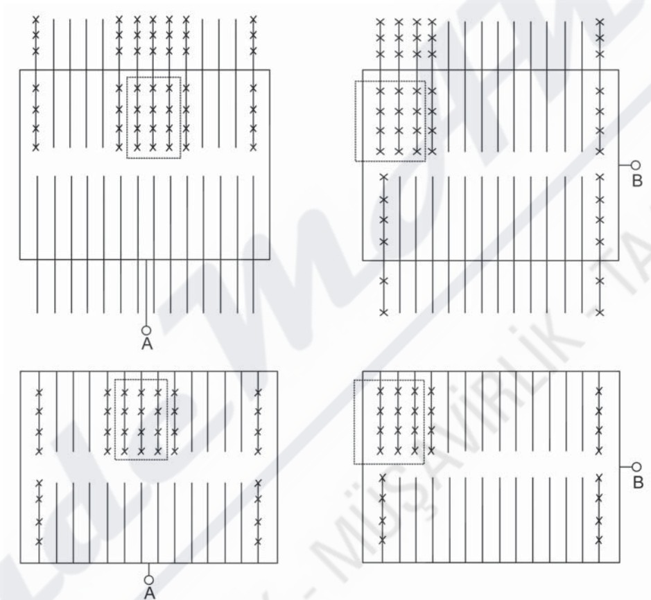
Şekil 7.4.3.2(a) Kritik Hidrolik Tasarım Alanı Örnekleri
