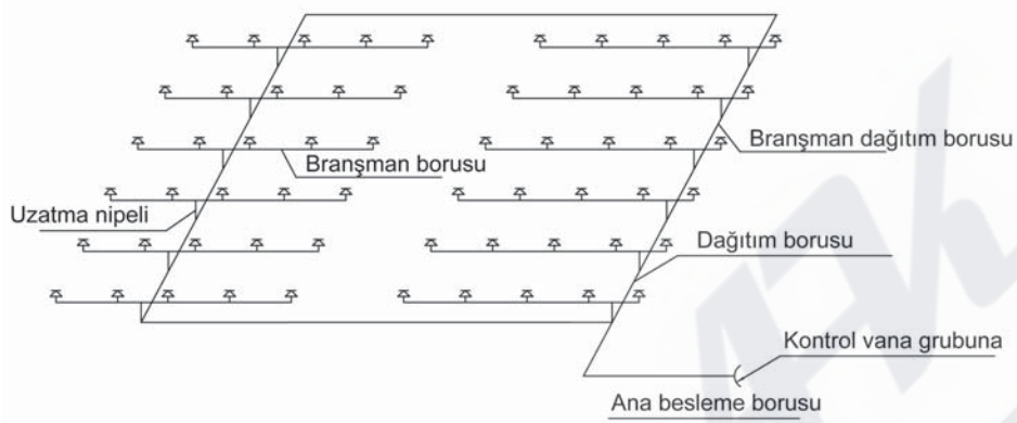
Şekil 7.2.2 Loop Borulama Sistemi
