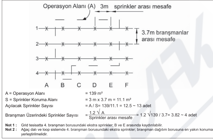
Şekil 7.4.3.3 Örnek: Operasyon Alanında Açılacak Sprinkler Sayısının Hesabı
