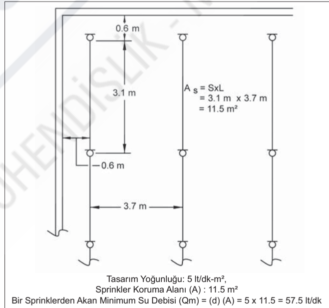
Şekil 7.4.3.5 Örnek: Bir Sprinklerden Akan Minimum Su Debisinin Hesabı
