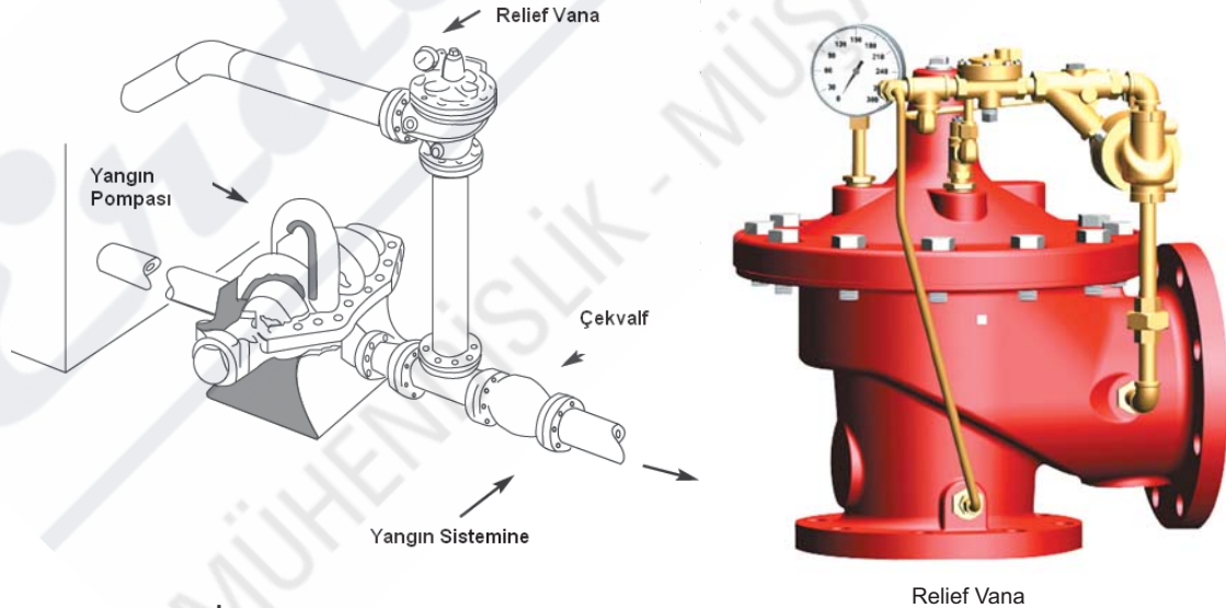
Şekil 8.9 Pompa İstasyonu Relief Vana Yerleşimi
