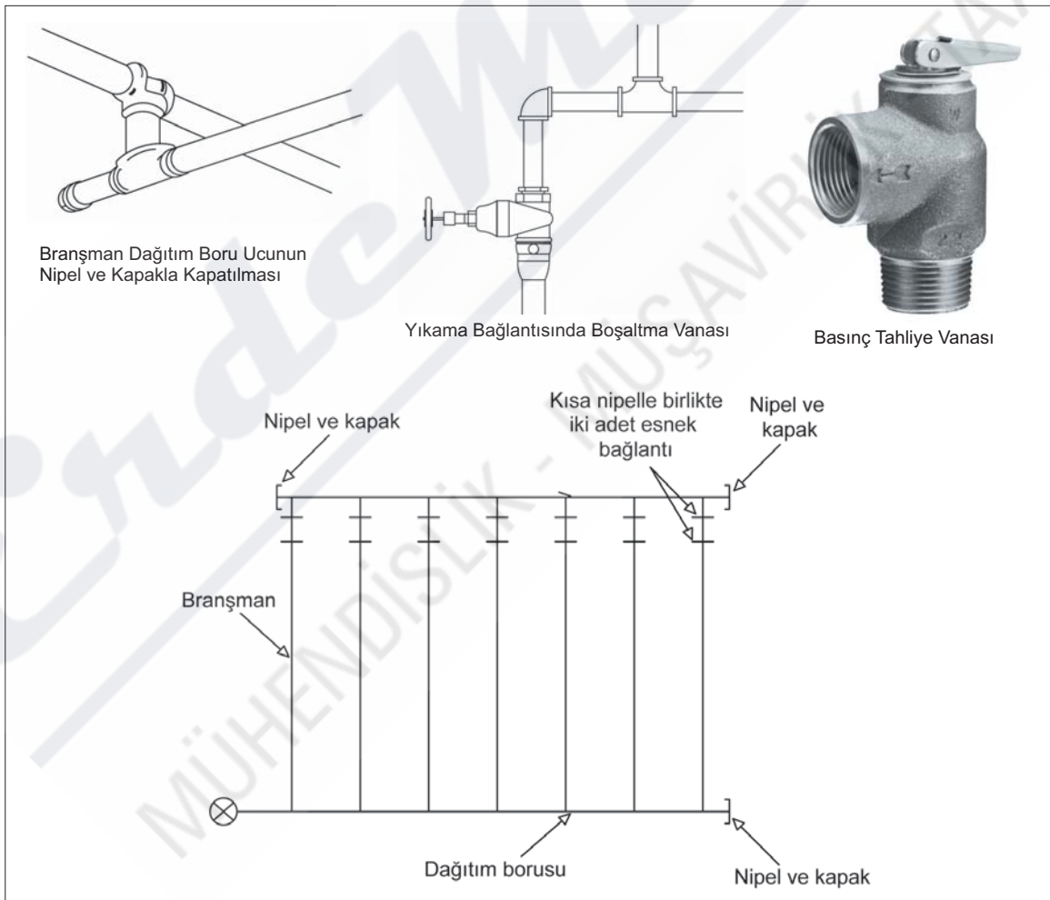
Şekil 8.11 Izgara Borulama Sisteminde Yıkama Bağlantısı Yerleşimi
