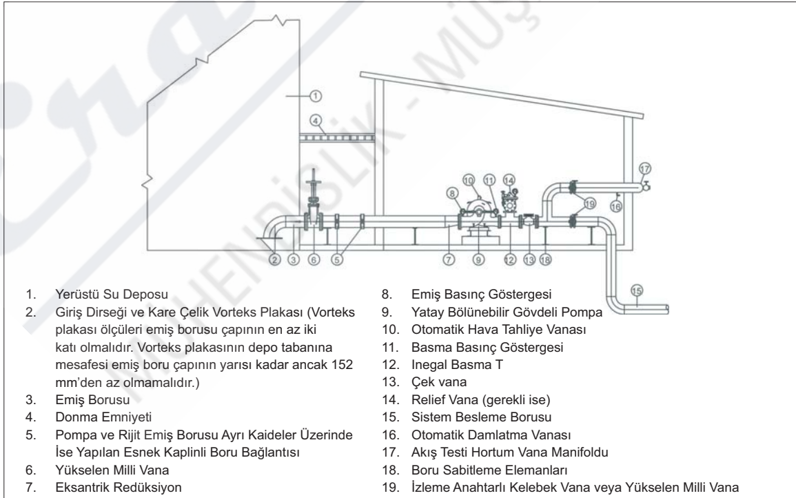
Şekil 8.20 Tipik Yangın Pompa İstasyonu
