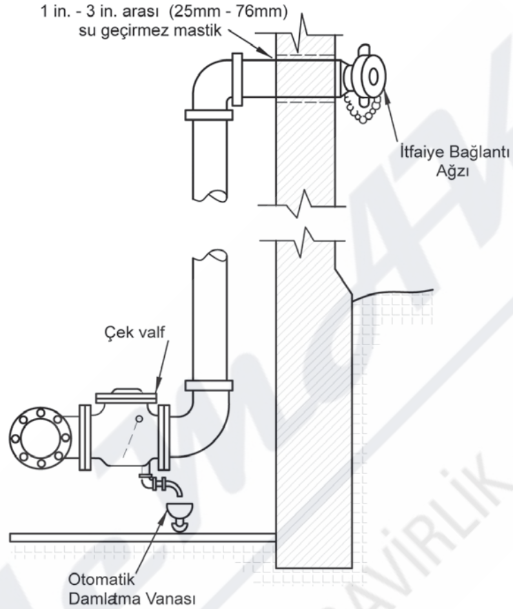
Şekil 8.16 İtfaiye Bağlantı Ağızı Yerleşimi
