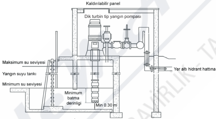
Şekil 8.19 Su Alma Bölmesi İçinde Dik Türbin Tip Pompa Yerleşimi
