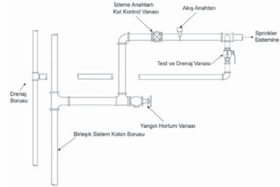
Şekil 8.3 (b) Birleşik Sistem Kat Vana Grubu
