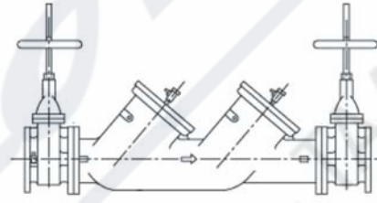
Geri Akış Önleyici
