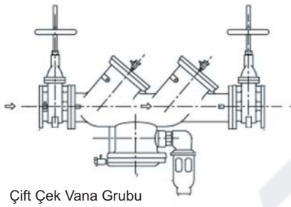
Çift Çek Vana Grubu
