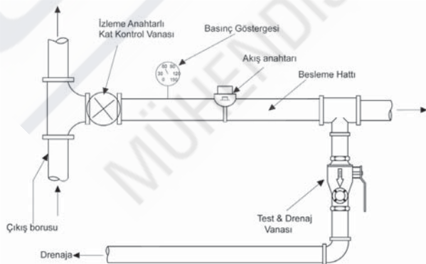
Şekil 8.3 (a) Islak Borulu Sprinkler Sistemi Kat Vana Grubu
