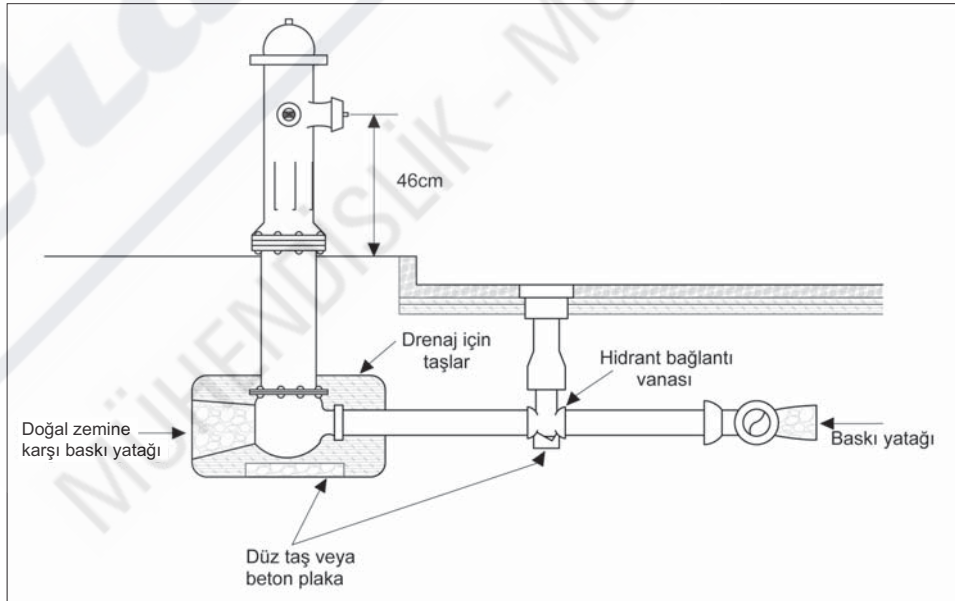
Şekil 8.13 Hidrant Yerleşimi
