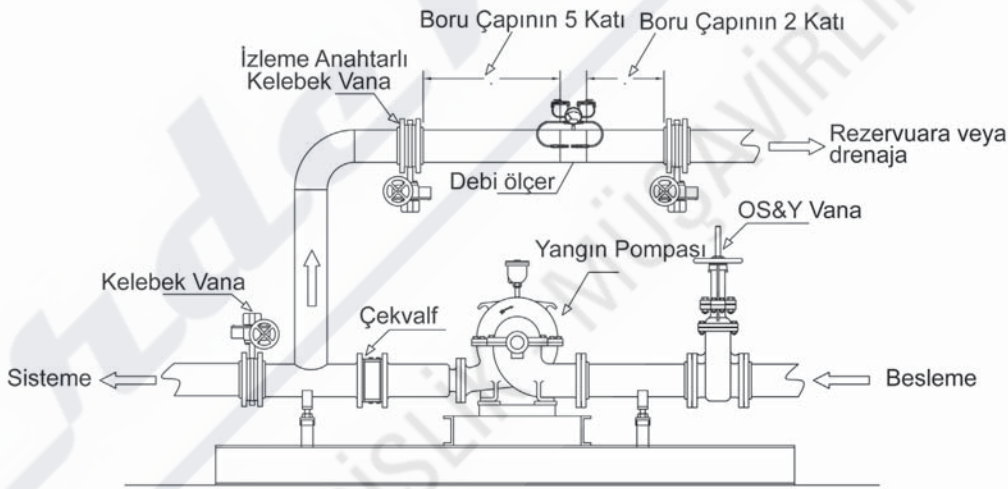
Şekil 8.17 Pompa Test Hattı
