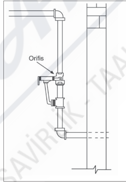
Şekil 8. 7 Kuru Borulu Sistemde Test ve Drenaj Vanası Yerleşimi
