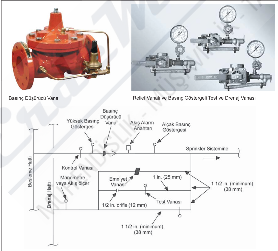
Şekil 8.10 Tipik Basınç Düşürücü Vana Hattı
