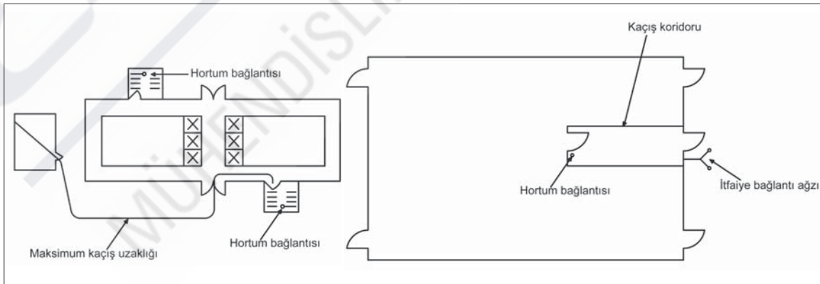
Şekil 8.15 Tipik Hortum Vanası Yerleşimi
