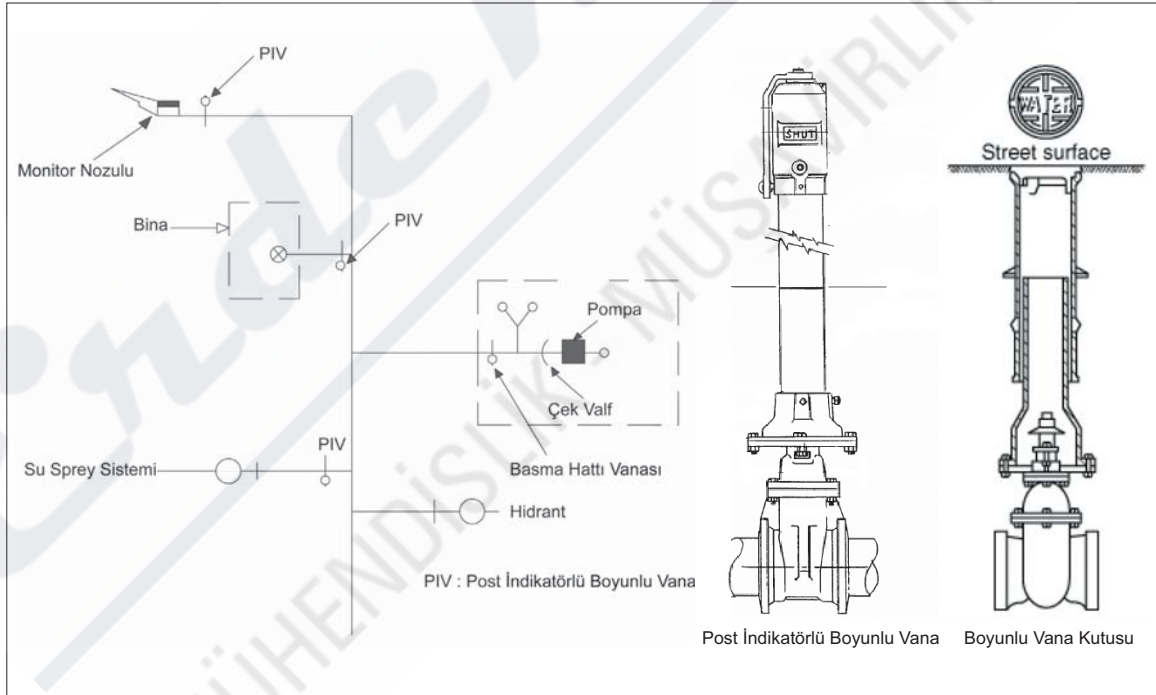
Şekil 8.2 Ana Yangın Besleme Hattı
